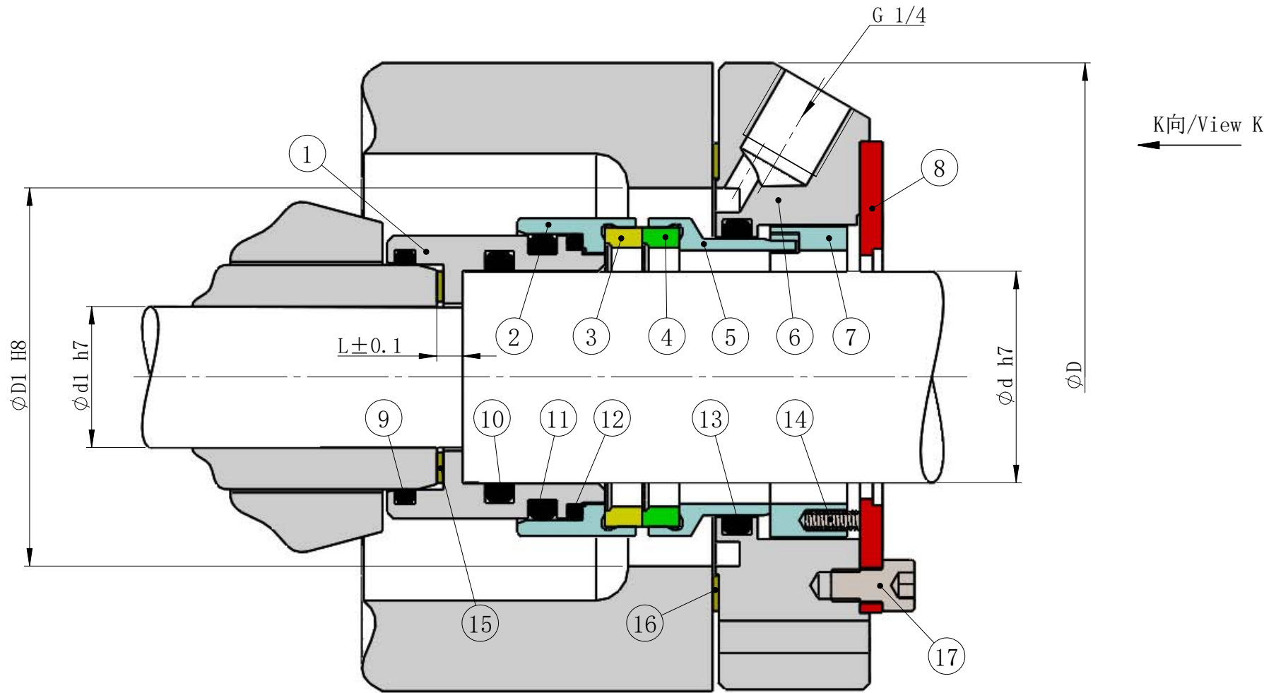
K向/View K 比例不符/NO SCALE
