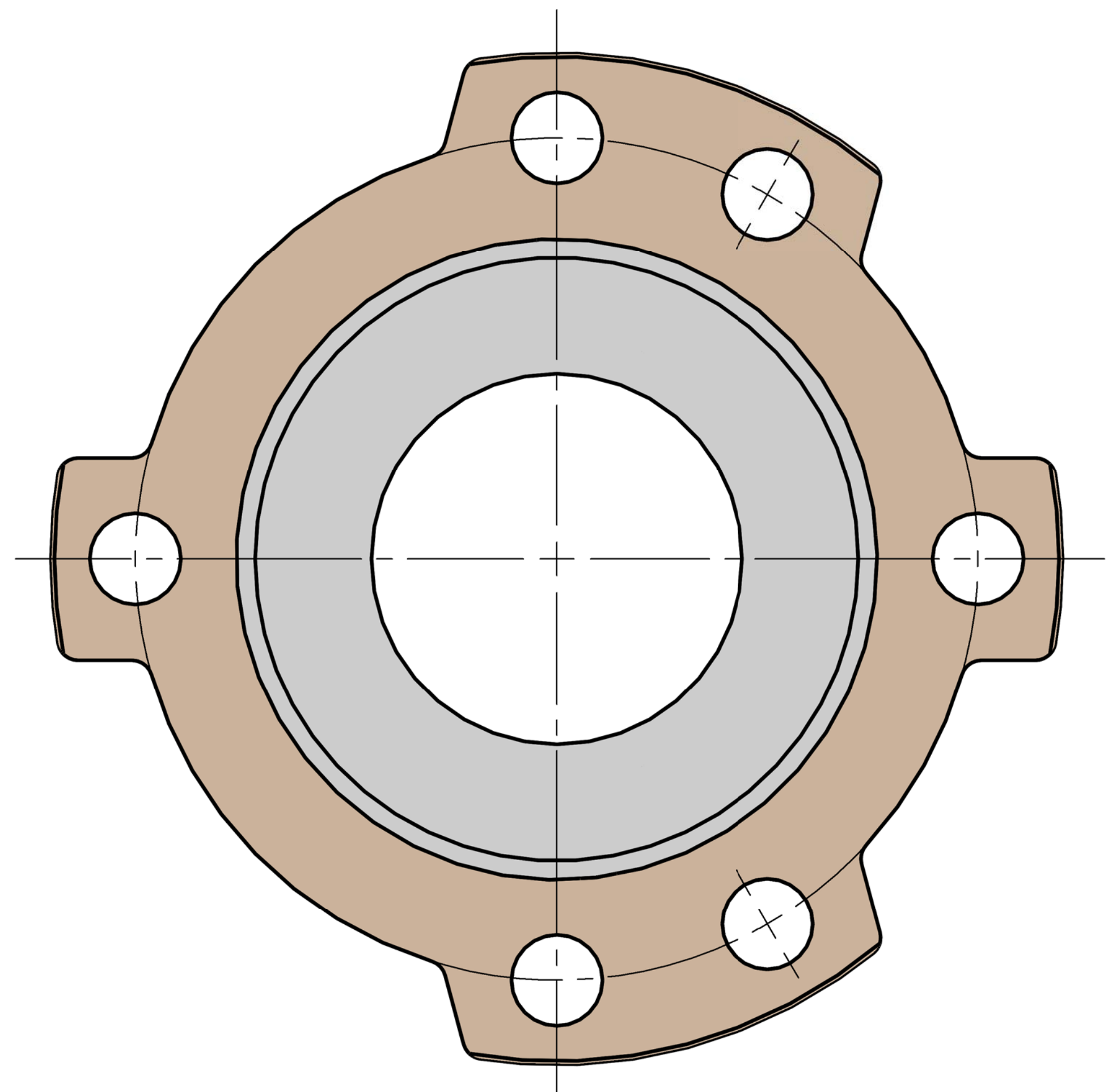
K向/View K 比例不符/NO SCALE
